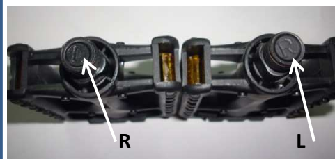
9.1. Colocación de los pedales. Considerando que estamos subidos en la bicicleta, el pedal con la letra R: se coloca a la derecha y rosca en sentido de las agujas del reloj.
